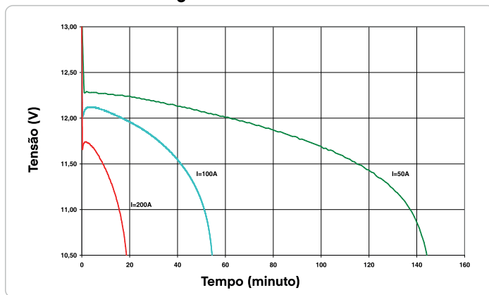
Curva de Descarga - Corrente Constante - DF 3000
