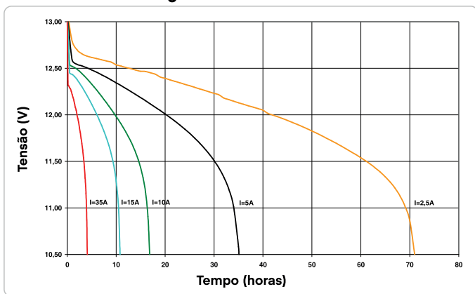
Curva de Descarga - Corrente Constante - DF 3000
